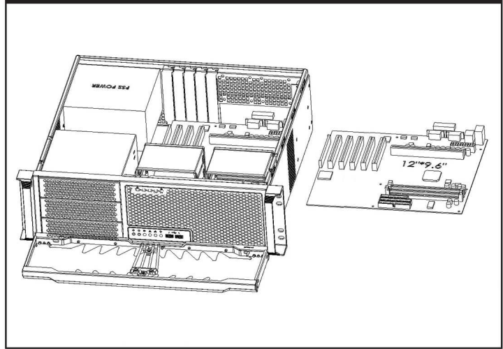
ATX MB / ATX主機板 / ATX ボード
